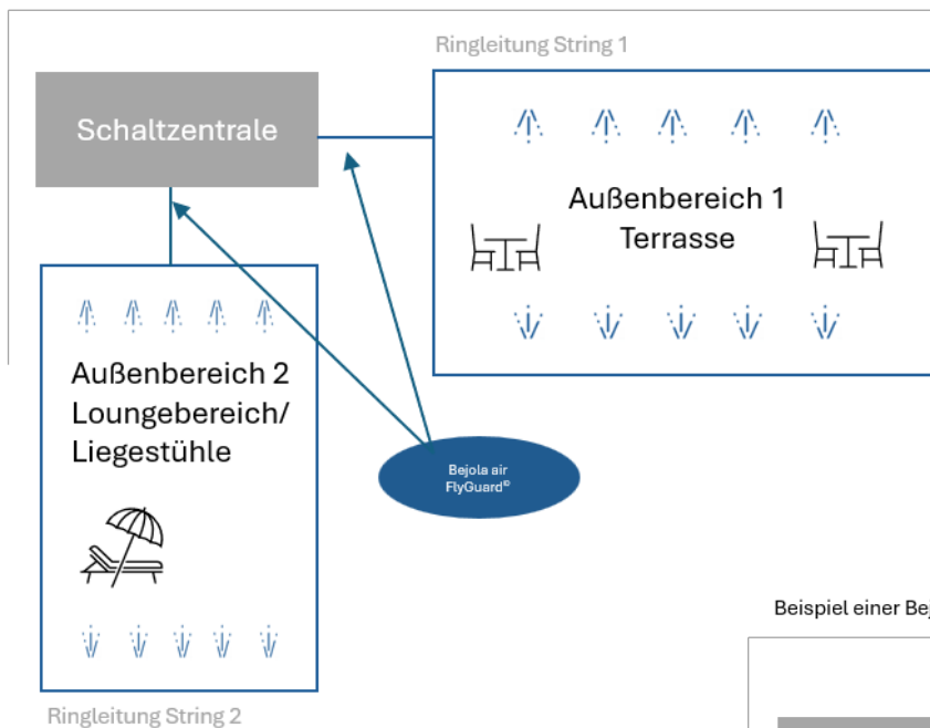
Beispiel einer Bejola 2-String-Sprühnebel-Anlage zwei Dosiereinheiten
