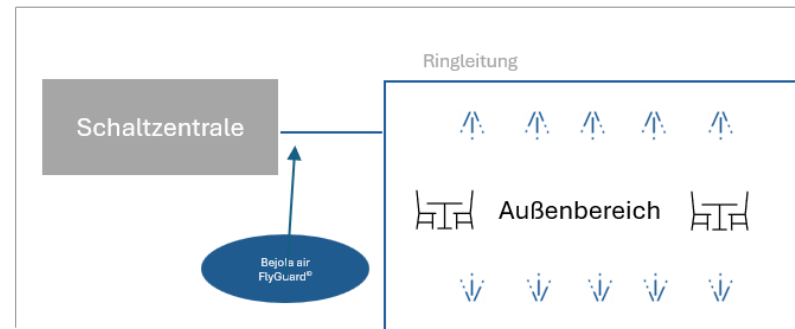
Beispiel einer Bejola 1-String-Sprühnebel-Anlage mit einer Dosiereinheit
